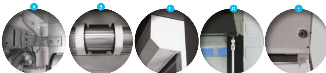
Gamme ENGADINE Tablier composé de lames de 77 x 19 mm
