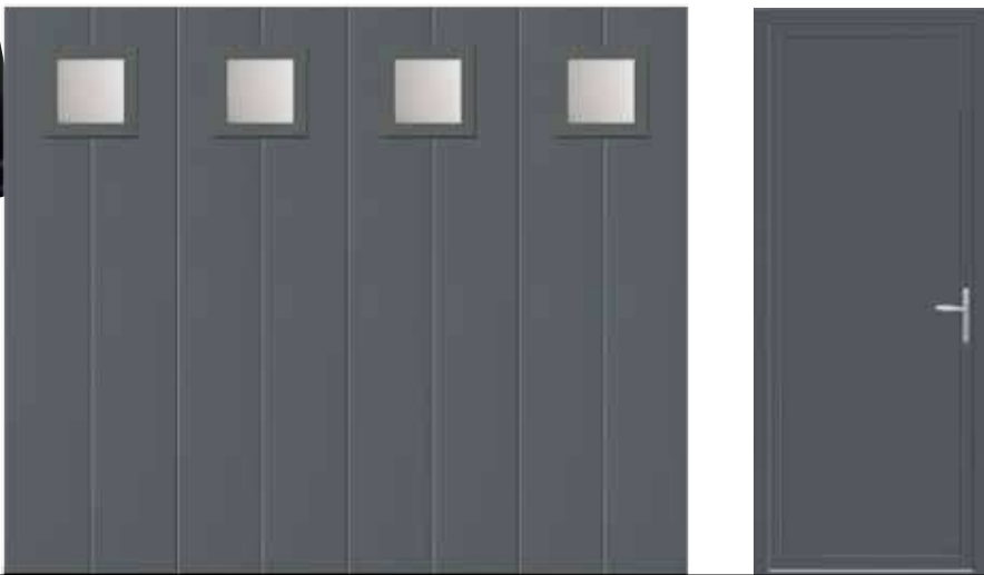
LOCARNO Porte de garage : RAL 7012 - Finition lisse Hublots carrés alu'nox laqués RAL 7012 Porte de service aluminium : RAL 7012 - Sans oculus Remplissage lisse de 24 mm La poignée existe en noir, blanc ou alu'nox (F9)
